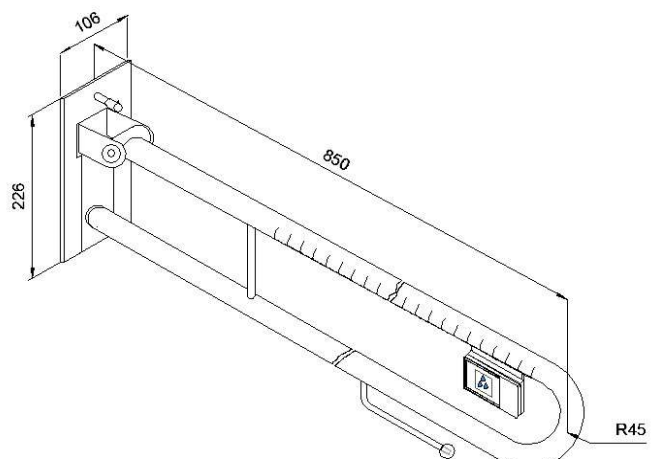
technische Zeichnung
